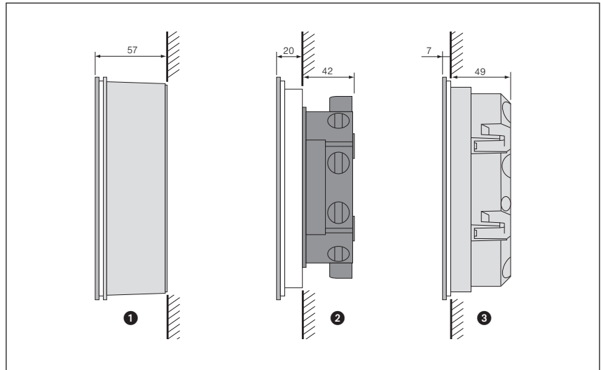
Abb. 6 Montagemöglichkeiten
