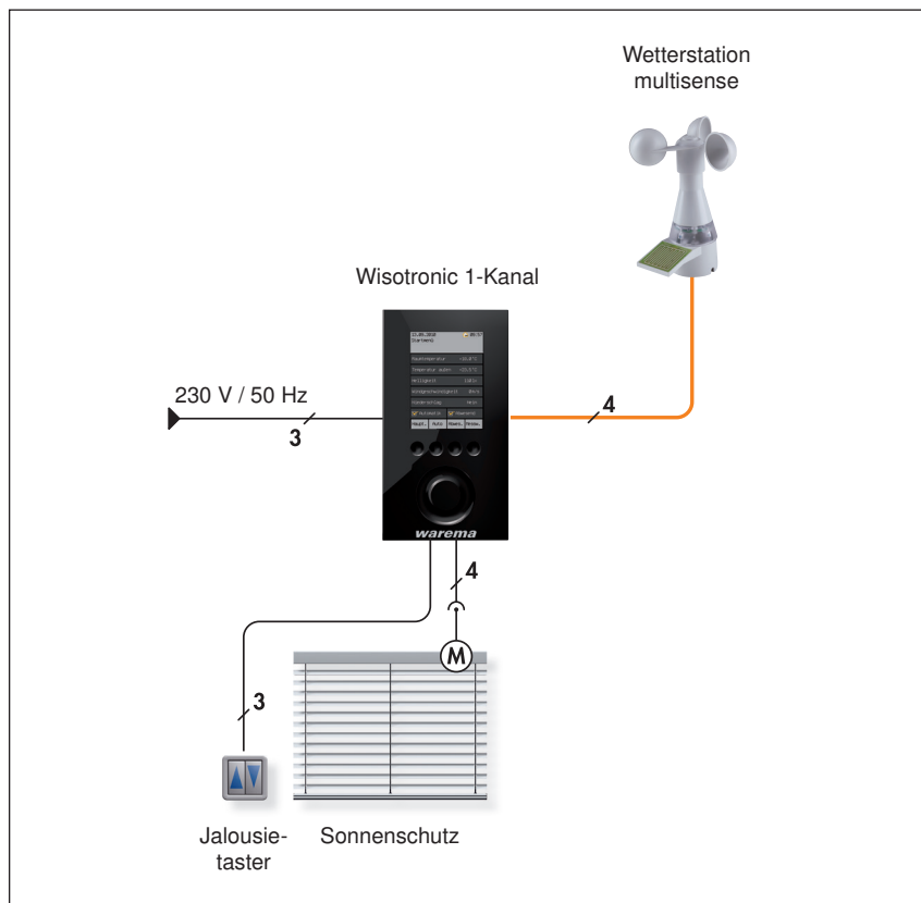
Abb. 2 Überblick über den Aufbau eines Wisotronic Systems
