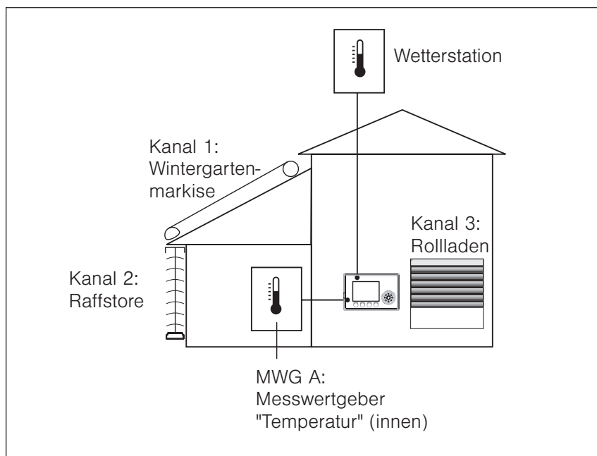
Abb. 16 Temperatursautomatik, Anwendungsbeispiel
