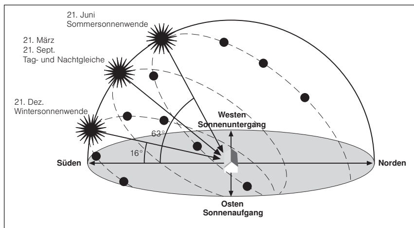
Abb. 12 Sonnenstand zu verschiedenen Jahreszeiten
