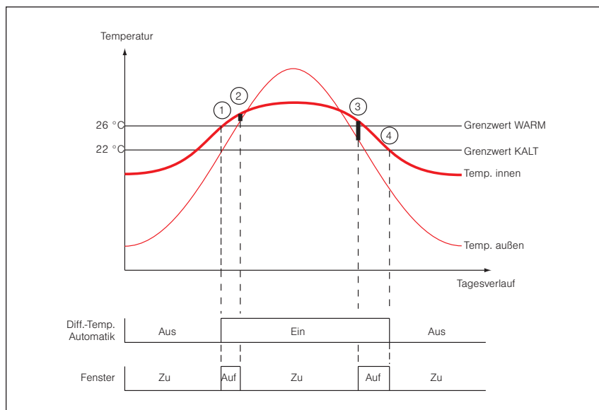
Abb. 17 Differenztemperaturautomatik
