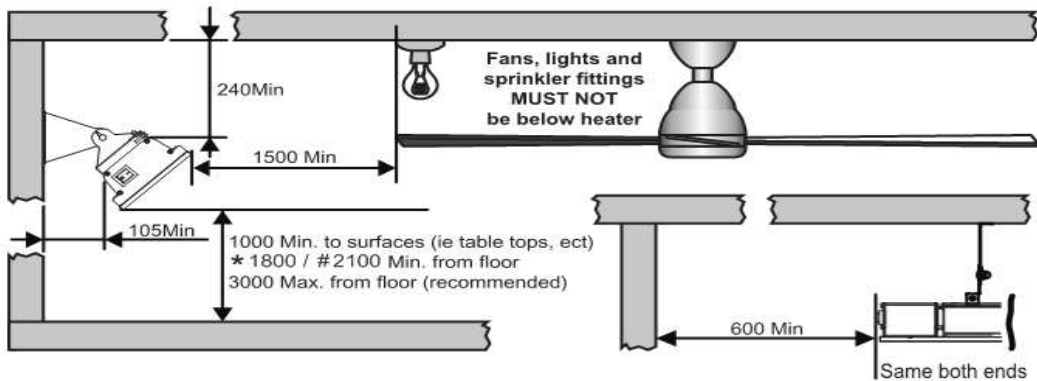
Mindestabstände bei Montage des Heizgeräts an einer VERTIKALEN WAND
