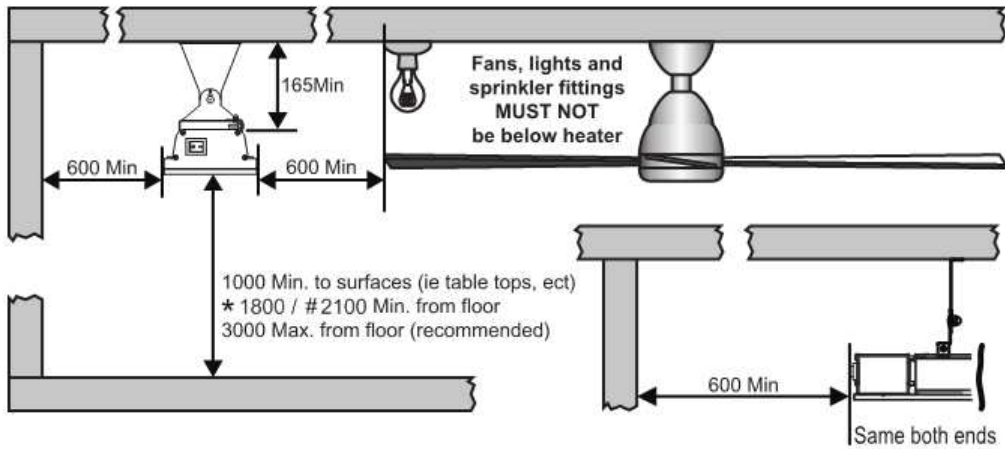
Mindestabstände bei Montage des Heizgeräts schräg zur Decke
