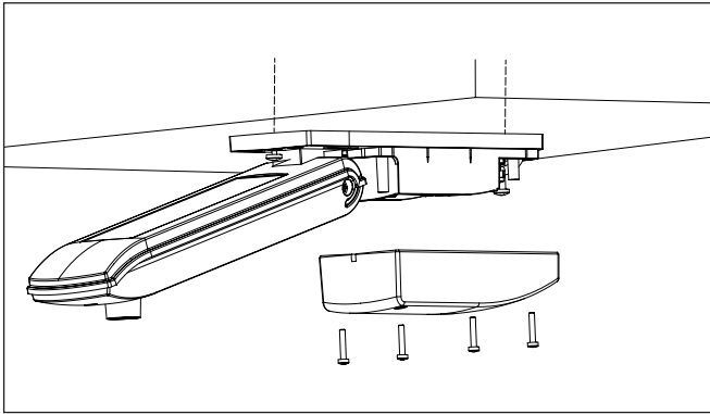
Abb. 5 Deckenmontage
