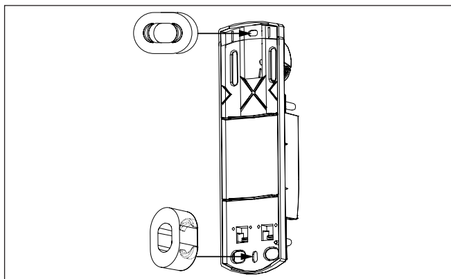
Abb. 2 Einclippen der separaten Abstandhalter ins Schraubloch
