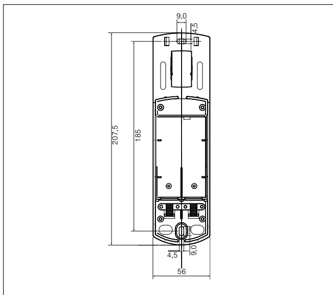
Abb. 3 Abmessungen
